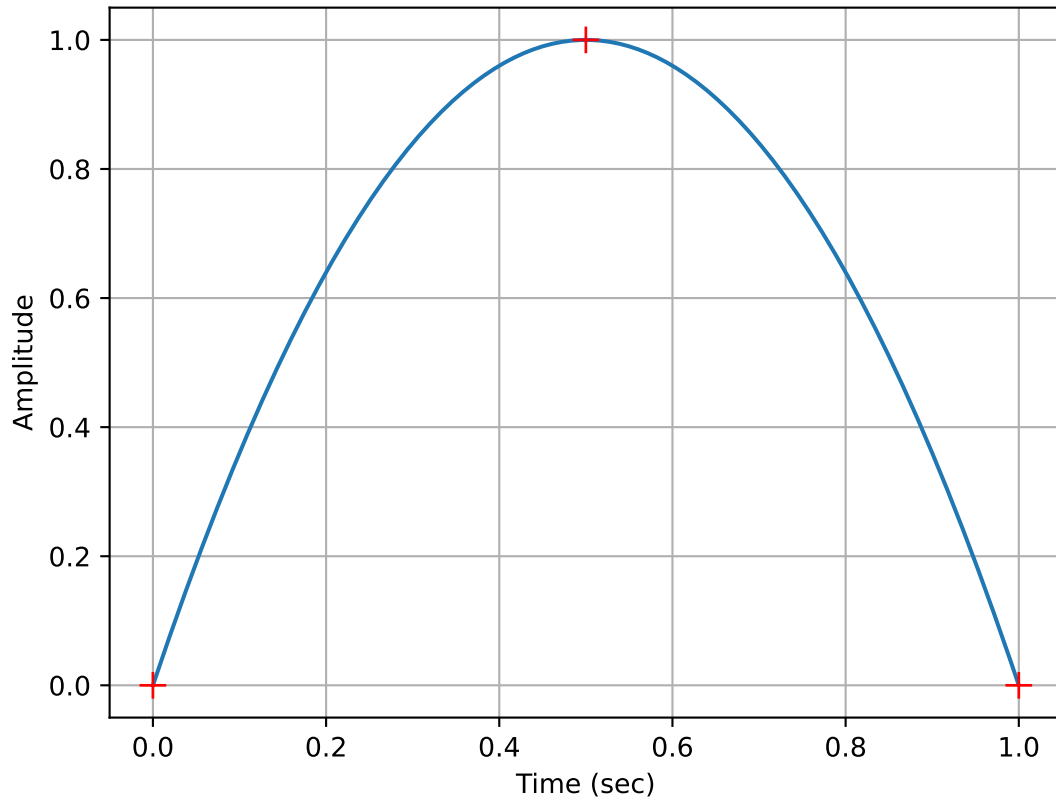
A Parabola
